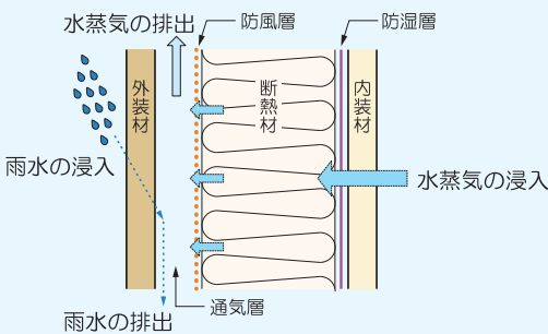
断熱壁体の構成
